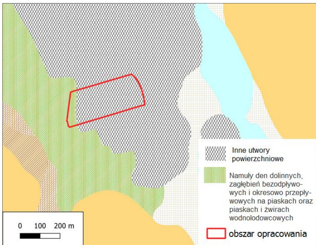
Rysunek 8. Fragment Szczegółowej Mapy Geologicznej Polski 1:50 000
