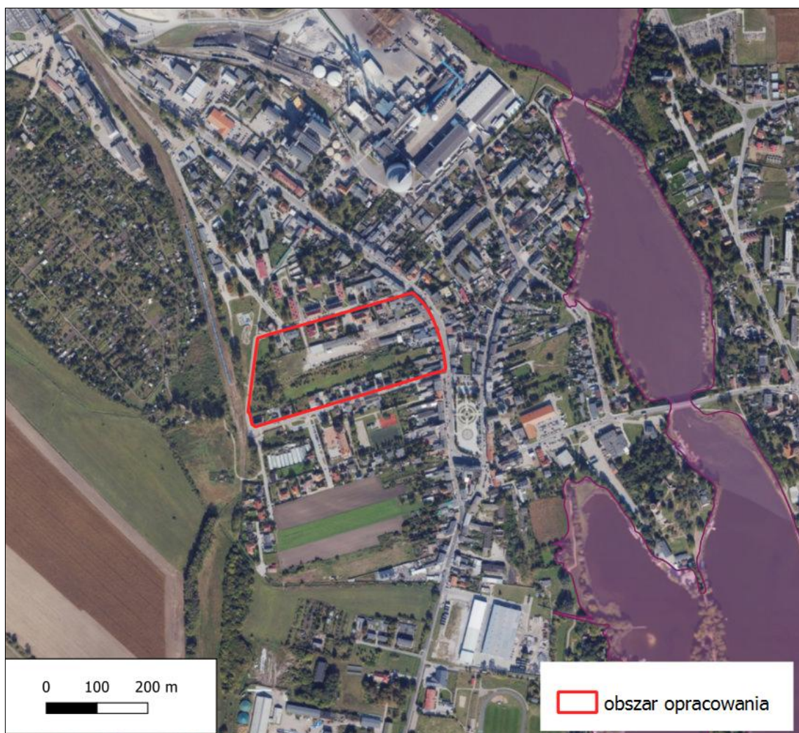
Rysunek 18. MZP z głębokością wody 10% (raz na 10 lat)
