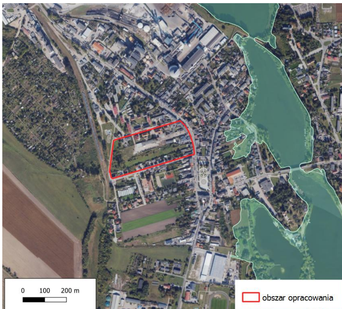
Rysunek 17. MZP z głębokością wody 0,2% (raz na 500 lat)
