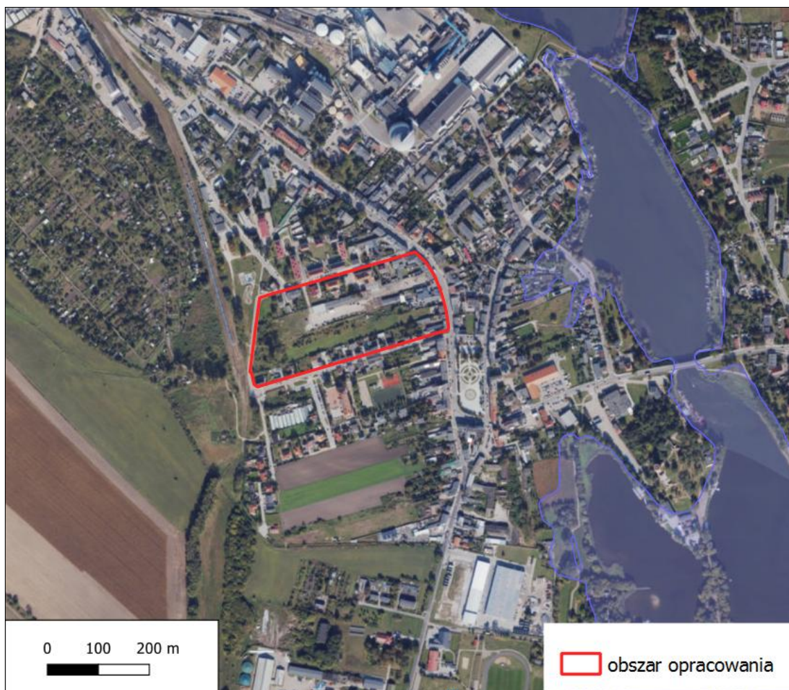
Rysunek 16. MZP z głębokością wody 1% (raz na 100 lat)
